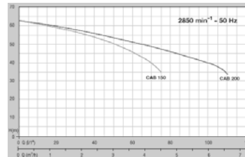
PENTAX-CAB پمپ های خود مکش مجهز به دو پروانه
