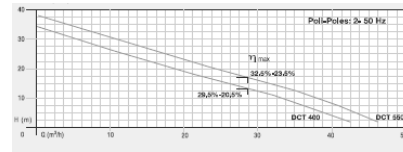
PENTAX-DC پمپهای مستغرق کفکش
