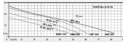
PENTAX-DM پمپهای مستغرق کفکش لجنکش تک کاناله
