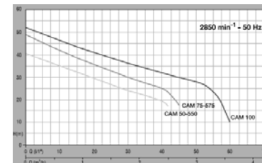
PENTAX-CAM پمپ های خود مکش مجهز به یک پروانه
