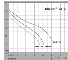
PENTAX-JMC پمپ های خود مکش مجهز به یک پروانه
