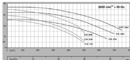
PENTAX-CH پمپهای سانتریفوژ مجهز به يك پروانه
