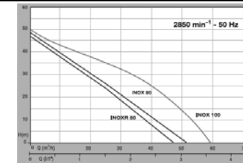
PENTAX-INOX پمپ های خود مکش مجهز به یک پروانه
