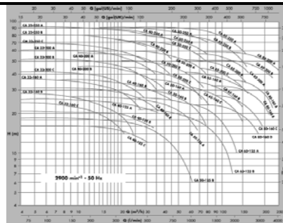
PENTAX-CA پمپهای سانتریفوژ یک طبقه
